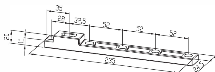
9123L Door strap
