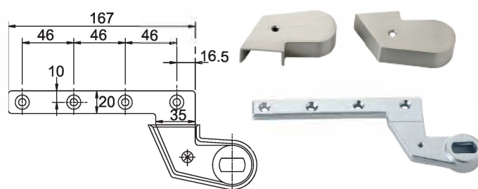
9149DS Offset Door strap
