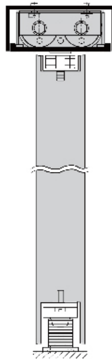
Double action timber door
